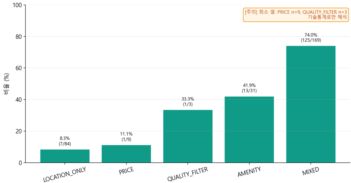
그림 4. A2 검색의도별 결과 없음률
