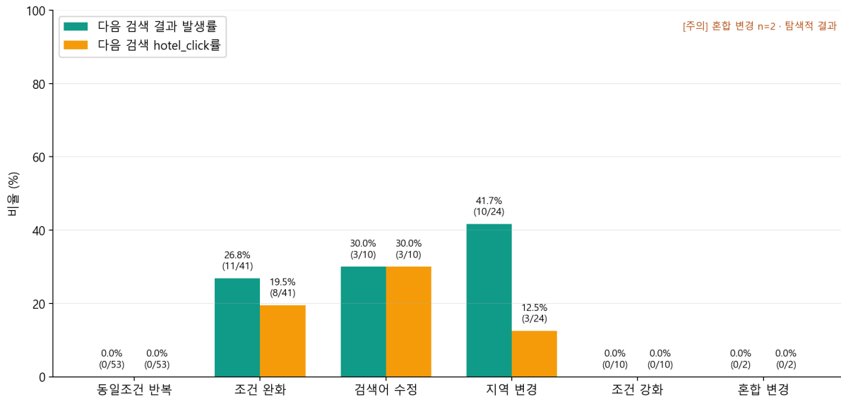
H3 — 재검색 유형별 다음 검색 결과
